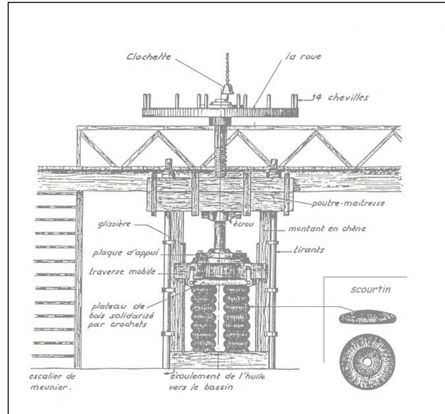
Croquis du pressoir
