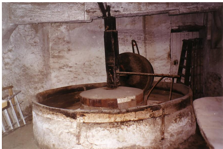
Vue d'ensemble du broyeur
