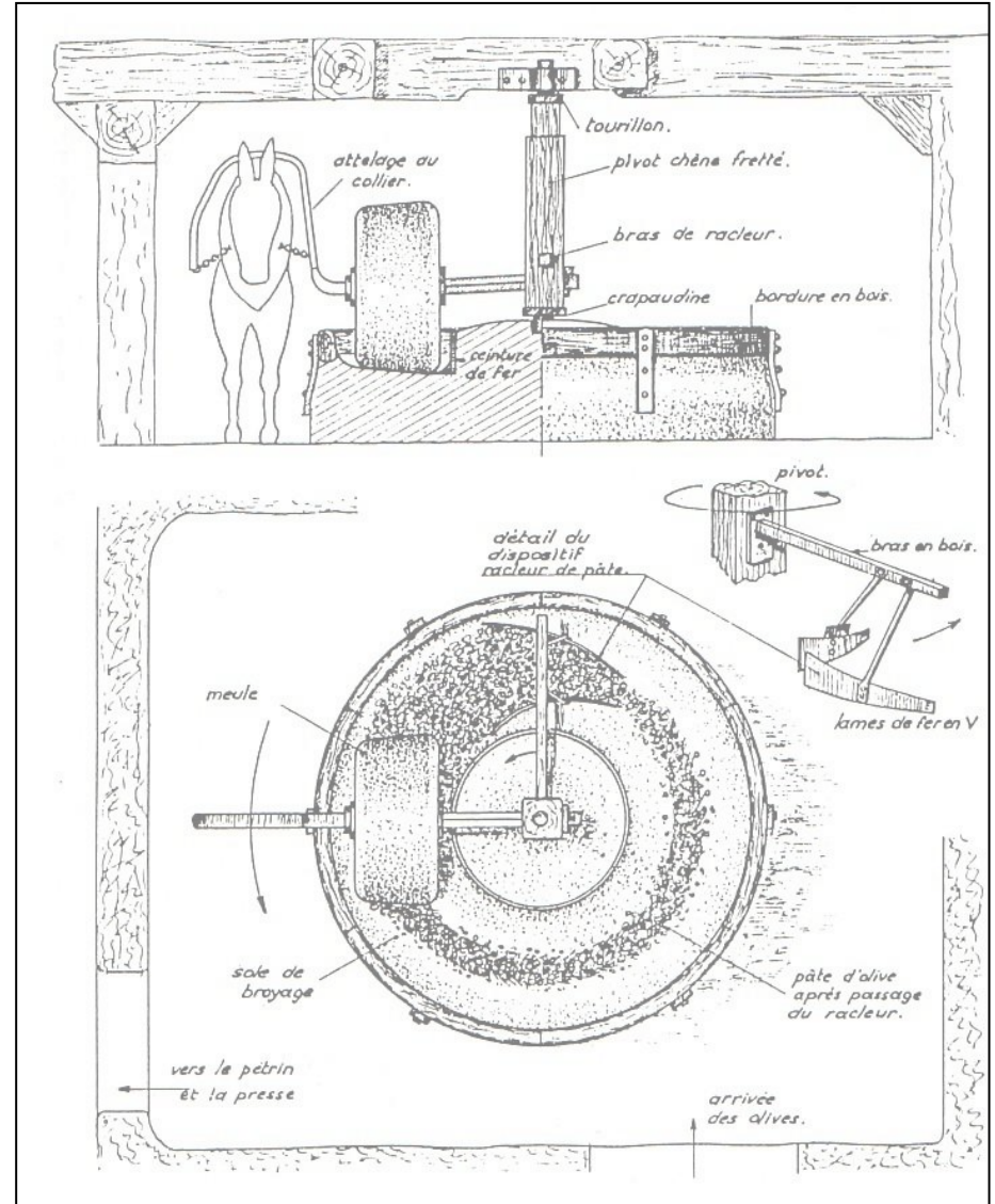
Croquis du broyeur
